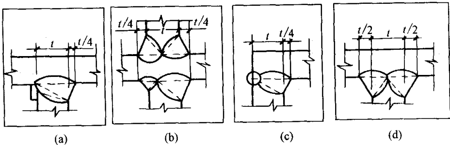
图 5.2.5 焊脚尺寸
